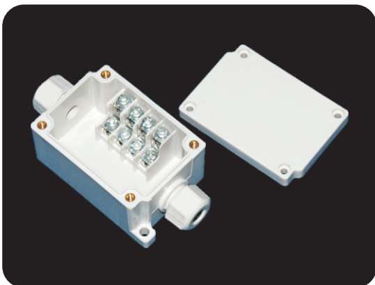
型号 (Model): TJ-4P 尺寸 (Size): 50×102×40mm
