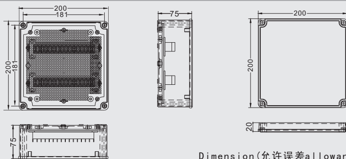
Dimension (允许误差 allowance \pm 1\text{mm} )
