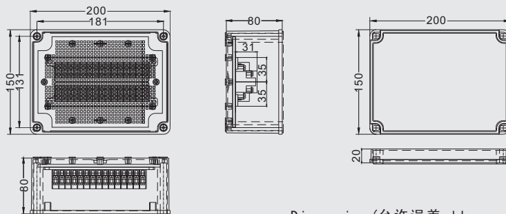
Dimension (允许误差 allowance \pm 1\text{mm} )
