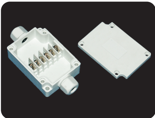
型号 (Model): PBT-6P 尺寸 (Size): 50×70×24mm
