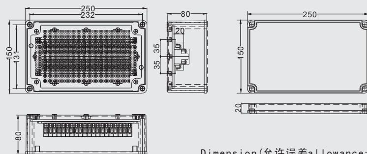
Dimension (允许误差 allowance \pm 1\text{mm} )
